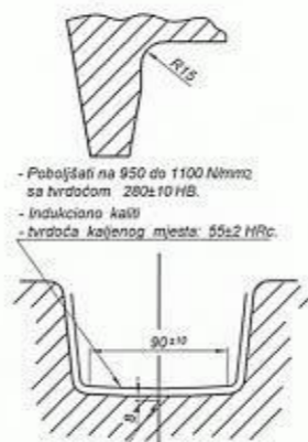
Presjek F - F
