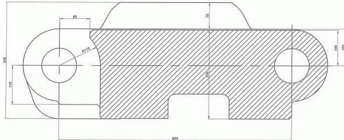
Presjek C - C
