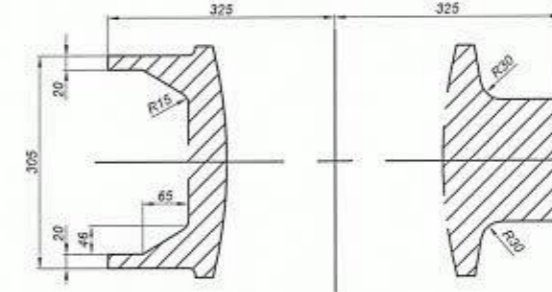
Presjek E - E (M-1.5)
